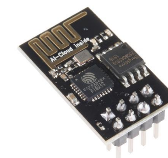
ESP8266 Wifi Module
